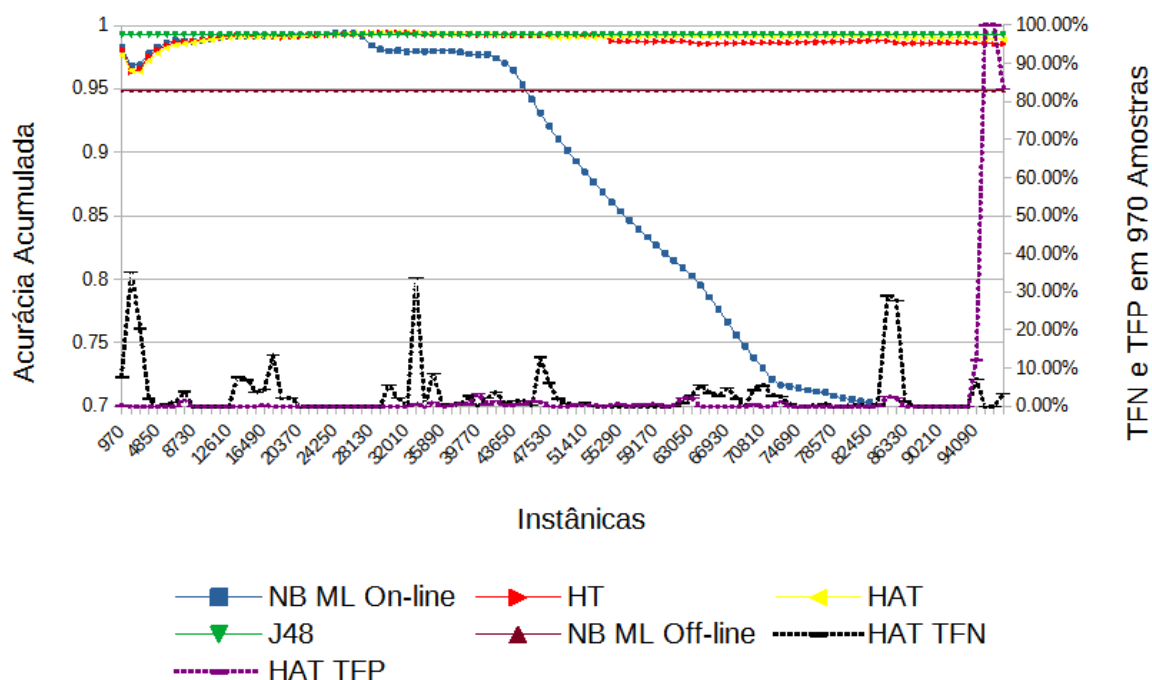
Figura 10: Acurácia do ML Off-line e ML On-line (eixo y principal), Taxa de Falso Negativo e Taxa de Falso Positivo do classificador Hoeffding Adaptive Tree do ML On-line em 970 amostras (eixo y secundário) do dataset Morris-3 gas.
